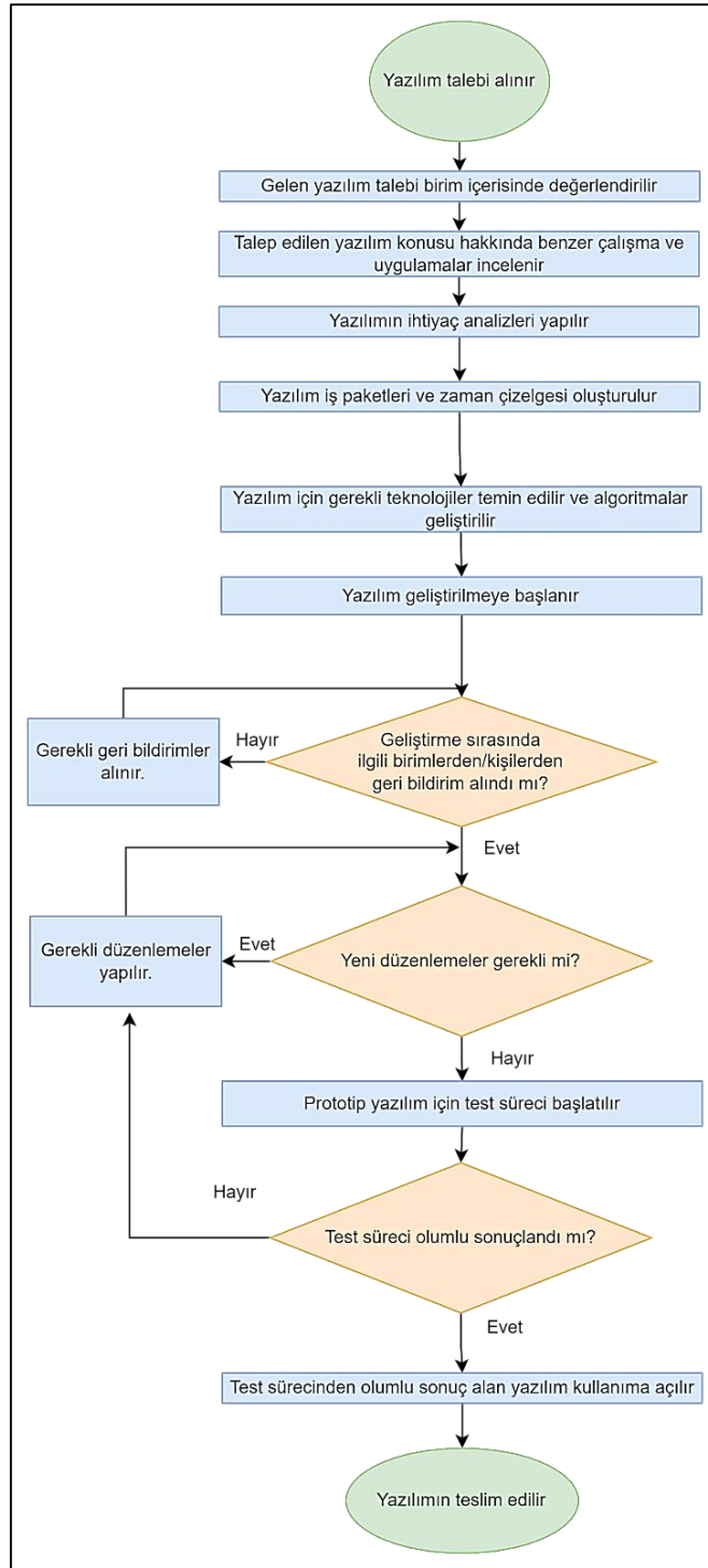
Şekil 1. Yazılım geliştirme süreci iş akış diyagramı
